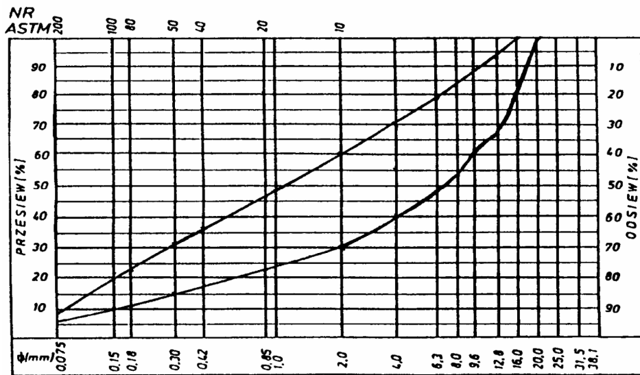
Rys. 1. Krzywe graniczne uziarnienia mieszanki mineralnej 0+20 mm do warstwy ściernalnej z betonu asfaltowego dla KR 1-2
