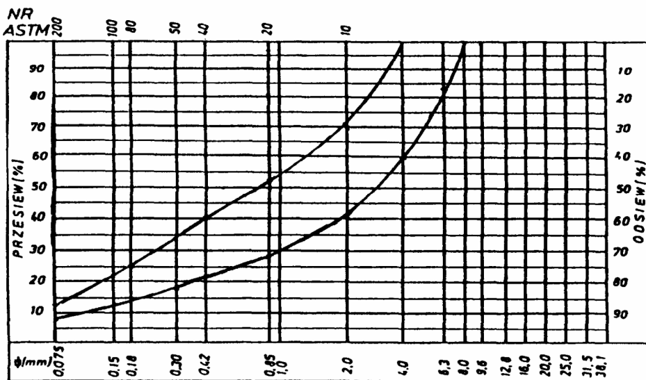
Rys. 3. Krzywe graniczne uziarnienia mieszanki mineralnej 0+8, 0+6,3 mm do warstwy ściernalnej z betonu asfaltowego dla KR 1-2
