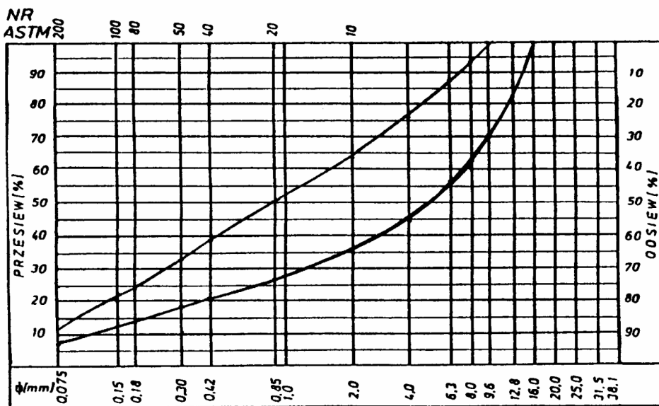
Rys. 2. Krzywe graniczne uziarnienia mieszanki mineralnej 0+16, 0+12,8 mm do warstwy ściernalnej z betonu asfaltowego dla KR 1-2
