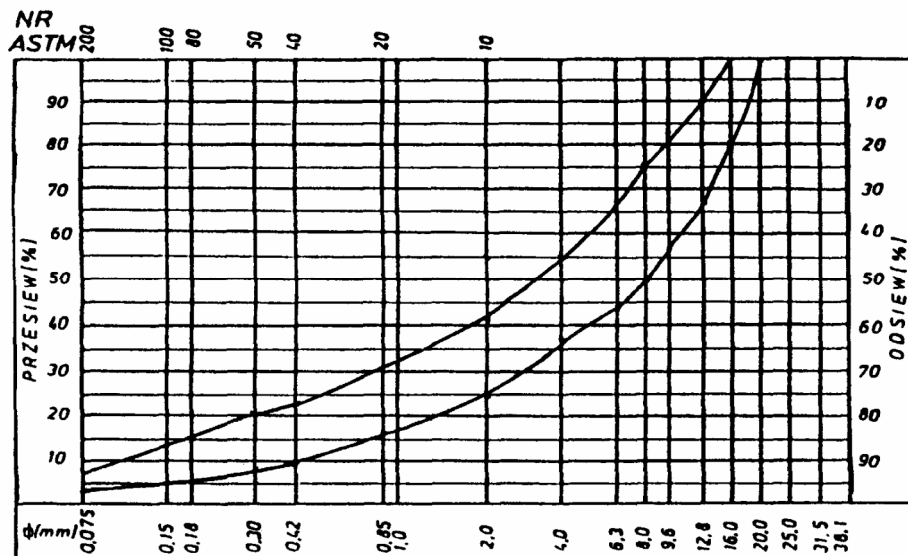
Rys. 11. Krzywe graniczne uziarnienia mieszanki mineralnej 0+25 mm do warstwy wiążącej, wyrównawczej i wzmacniającej z betonu asfaltowego dla KR 3-6
